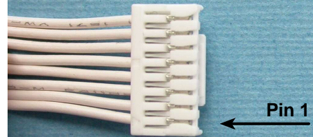
JST GHR-08V-S - 1.25 mm
